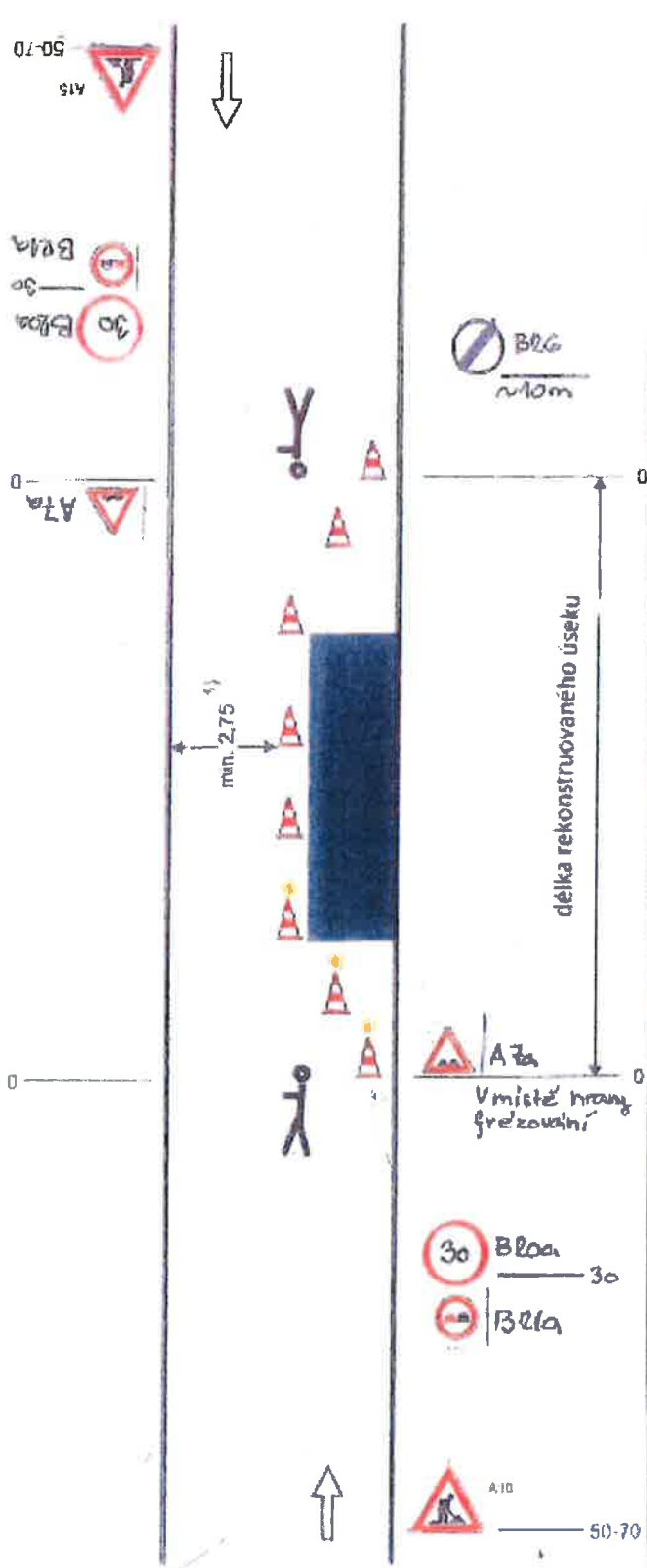
Označení pracovního místa během provádění oprav
